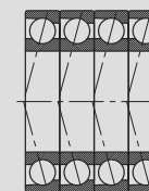
QTT Disposição em Tandem
