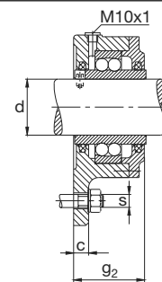
Execução F11209 e F11210
