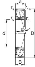
B719C, B70C Ângulo de contato \alpha = 15^\circ
