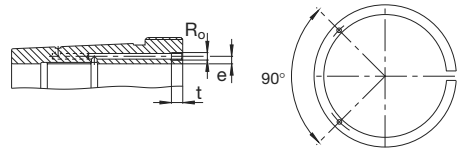
Buchas de desmontagem hidráulica (Sufixo H)
