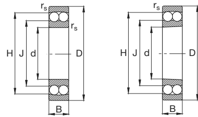
K Furo cônico (cone 1 : 12)
