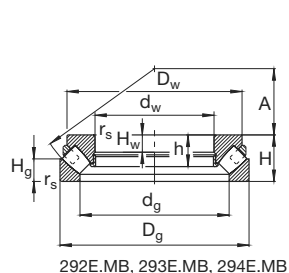
292E.MB, 293E.MB, 294E.MB
