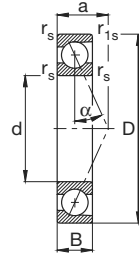
B719E, B70E Ângulo de contato \alpha = 25^\circ
