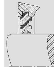
Vedação de dois lábios
