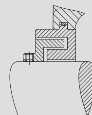
Vedação de labirinto axial
