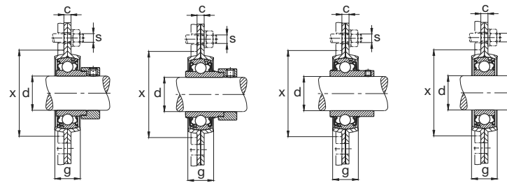
FBB2 Combinado com 162 FBB2 combinado com 362 FBB2 combinado com 562 FBB2 combinado com 762..2RSR
