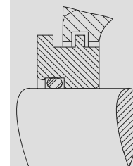
Vedação de labirinto radial
