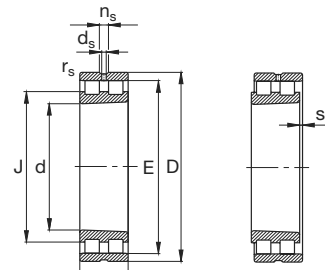
NN30ASK (conicidade 1:12)
